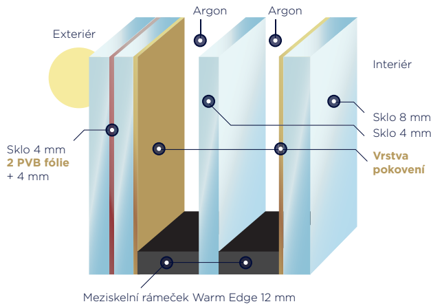
44.2 Si XN/12/4/12/8 XN | Stupeň zvukové izolace 45 dB
